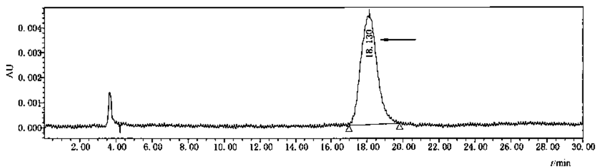
图 A.1 10 µg/mL 维生素 B 12 标准溶液色谱图(氨基柱)
