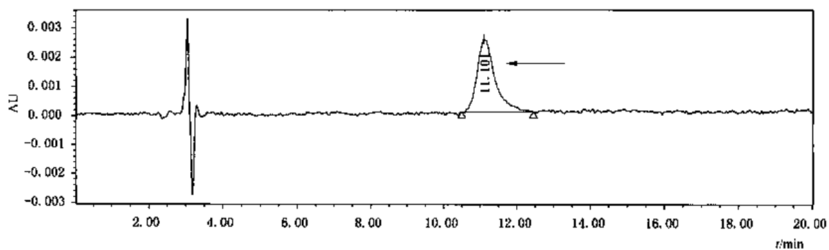
图 A.1 10 µg/mL 维生素 B 12 标准溶液色谱图(氨基柱)
